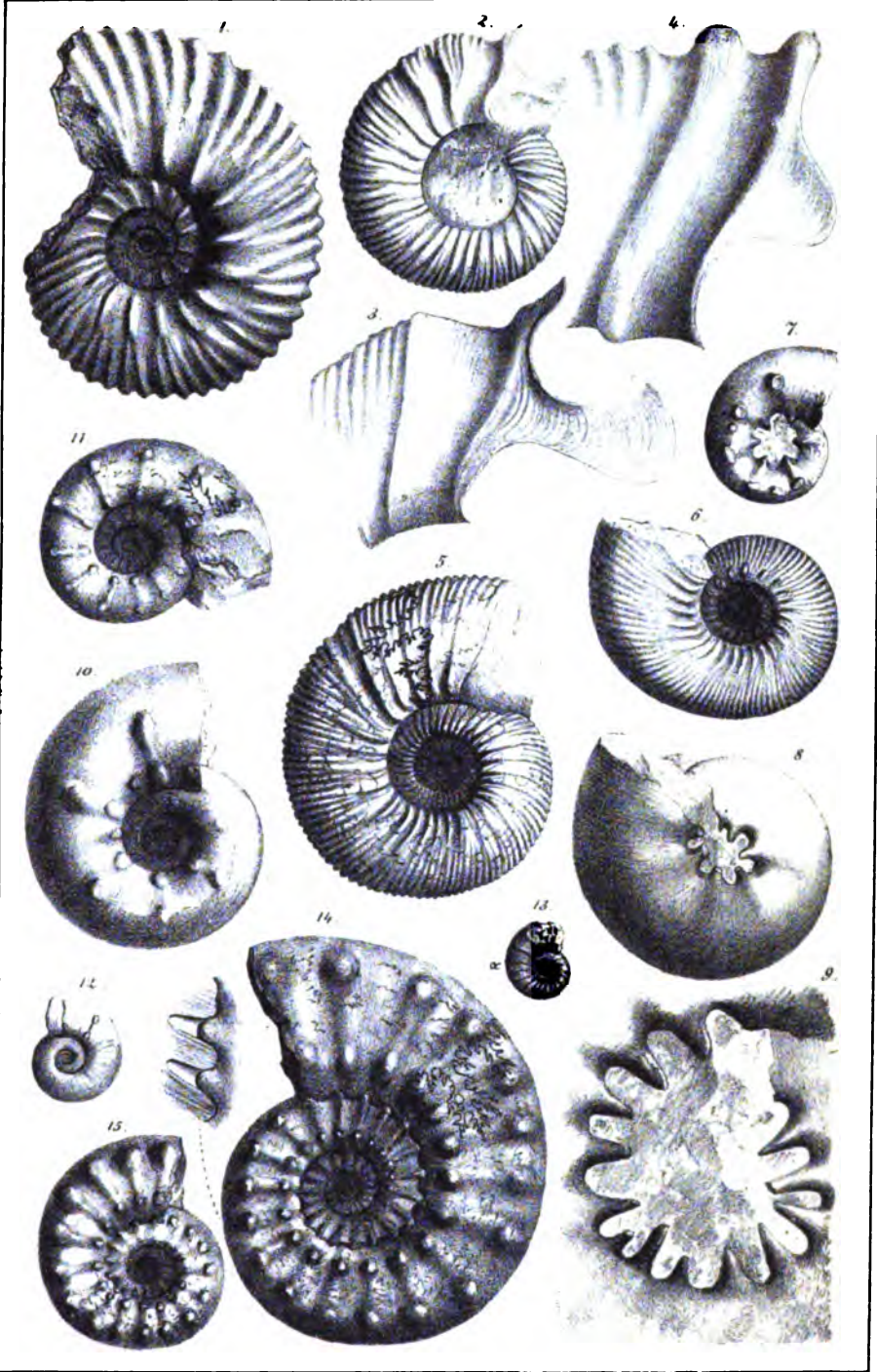
Auenstedt, iura.
